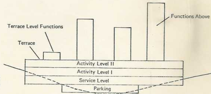
289 Schematischer Schnitt durch die Basisstruktur des Stadtkerns
